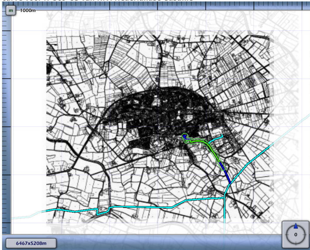
Figuur 4.2 Kilometer leiding behorende bij de maximale overschrijding van de FN-curve voor N-569-83 van N.V. Nederlandse Gasunie
