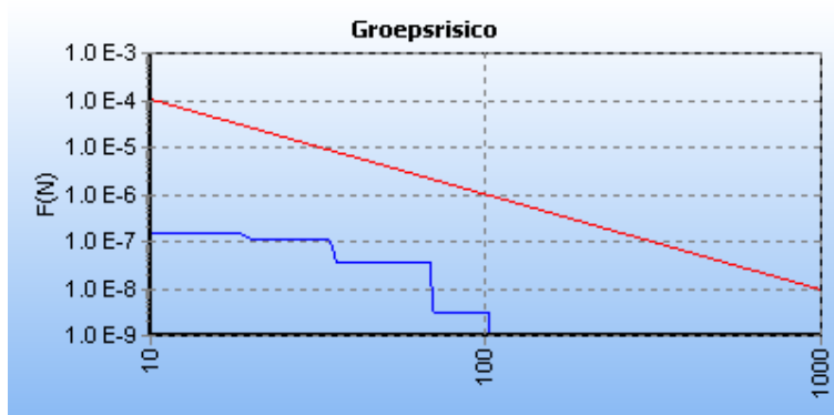
5.1 Figuur 5.1 FN curve voor N-569-83 van N.V. Nederlandse Gasunie voor de kilometer tussen stationing 500.00 en stationing 1500.00
